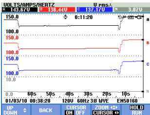
图 23-5. 趋势图显示（光标功能启用）
