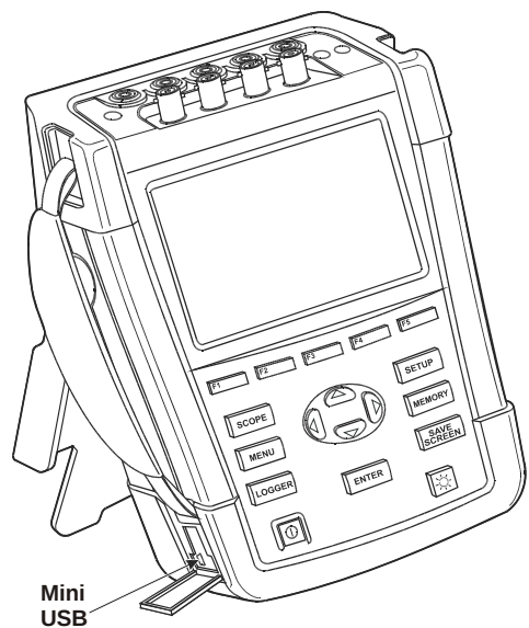
图 4-1. 仰角架与 USB 接口连接器的位置
