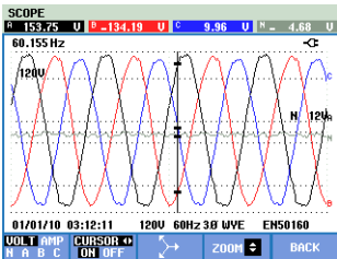
图 23-2. 波形显示（光标功能启用）
