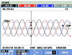
图 23-3. 波形显示（光标和缩放功能启用）
