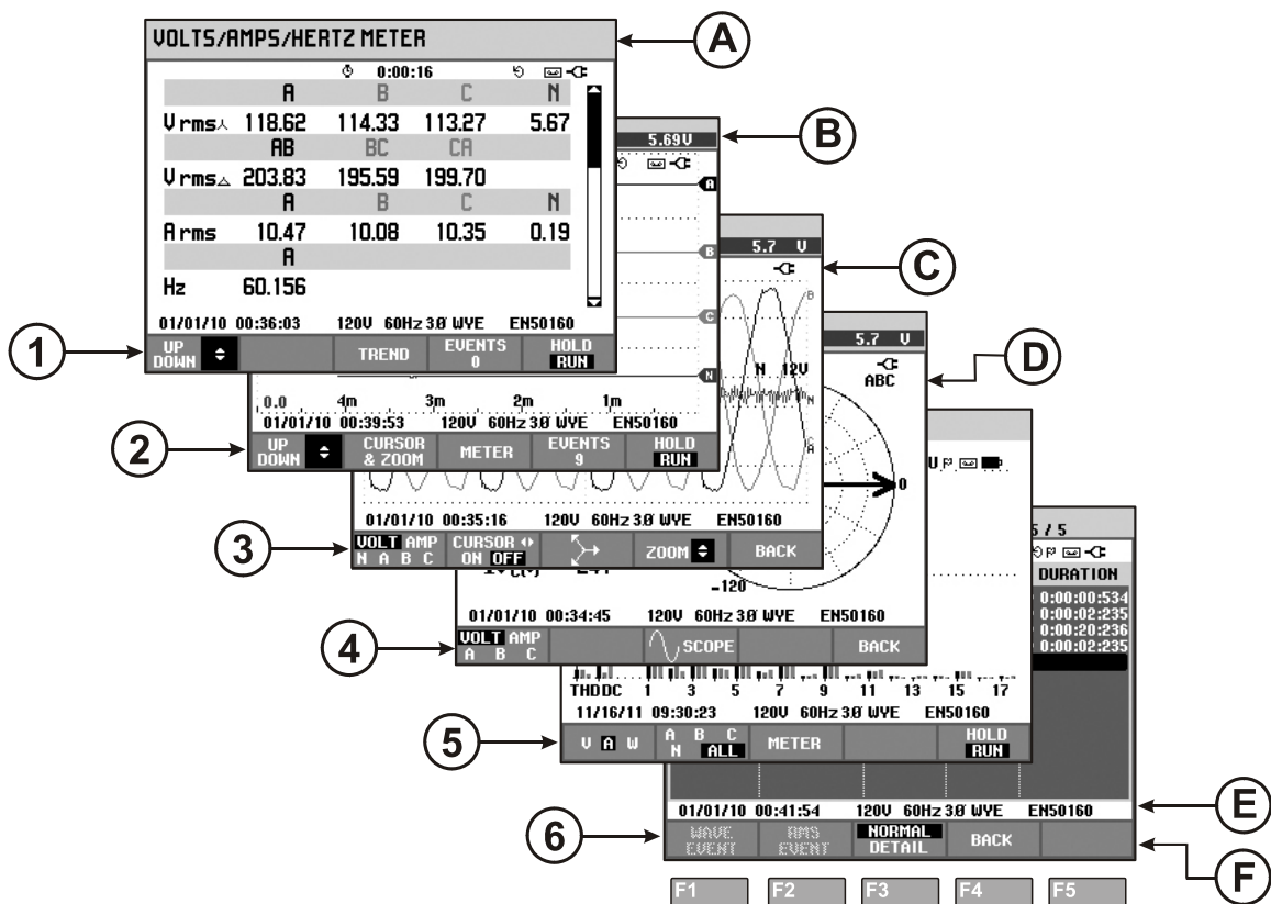
图 5-1. 显示类型概览
